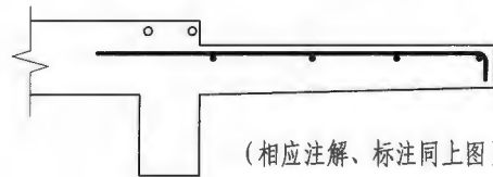
(仅上部配筋)
