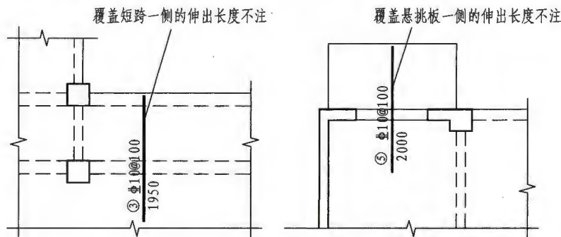
图 5.3.1-3 板支座非贯通筋贯通全跨或伸出至悬挑端
