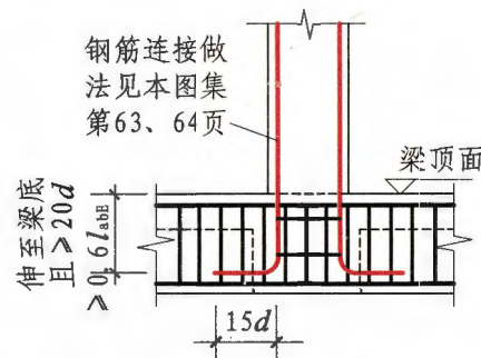
梁上柱LZ纵筋构造
