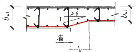
翼墙 (三)
