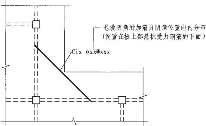
图 7.2.9 悬挑板阴角附加筋 C is 引注图示
