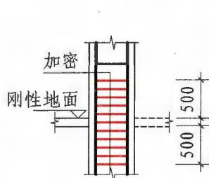
底层刚性地面前后上下各加密500
