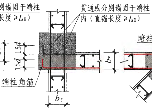
端柱翼墙 (三)
