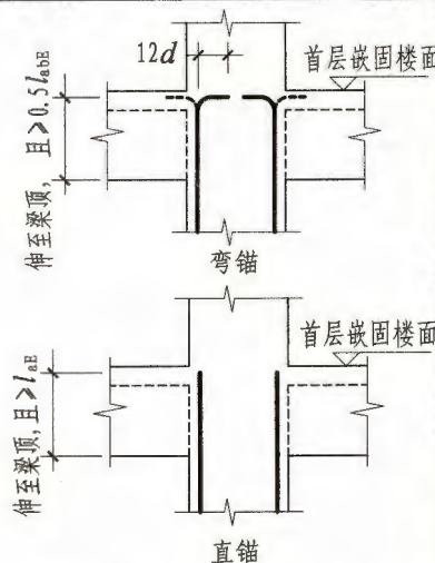
地下一层增加钢筋在嵌固部位的锚固构造
