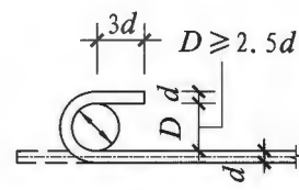
(a) 光圆钢筋末端180°弯钩
