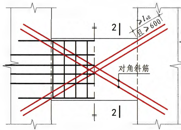
连梁集中对角斜筋配筋构造
