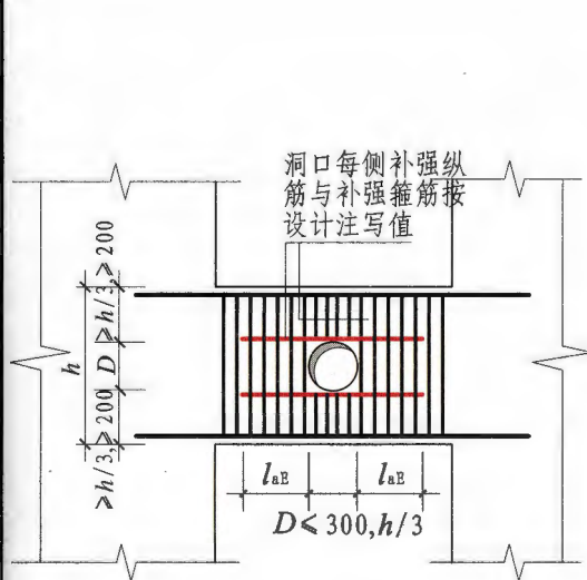
连梁中部圆形洞口补强钢筋构造
