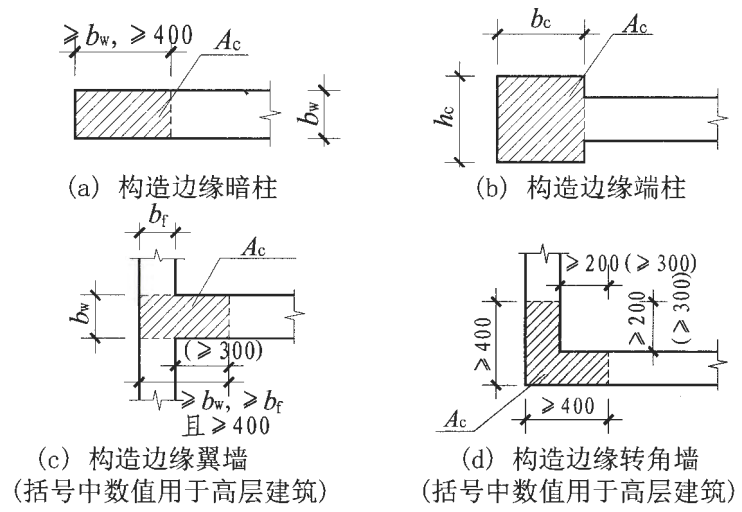
图 3.2.2-2 构造边缘构件
