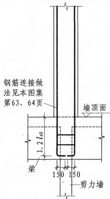
柱纵筋锚固在墙顶部时柱根构造
