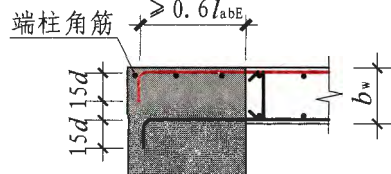
端柱端部墙 (二)
