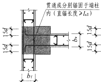
端柱翼墙 (一)
