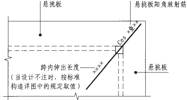
图 7.2.10-1 悬挑板阳角放射筋 C es 引注图示 (一)
