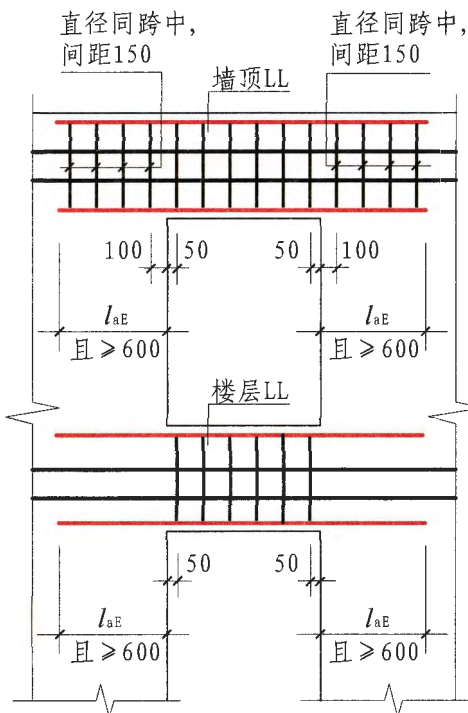
单洞口连梁 (单跨)
