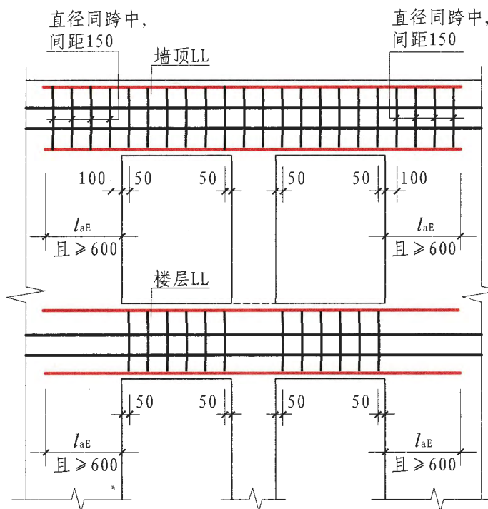
双洞口连梁 (双跨)
