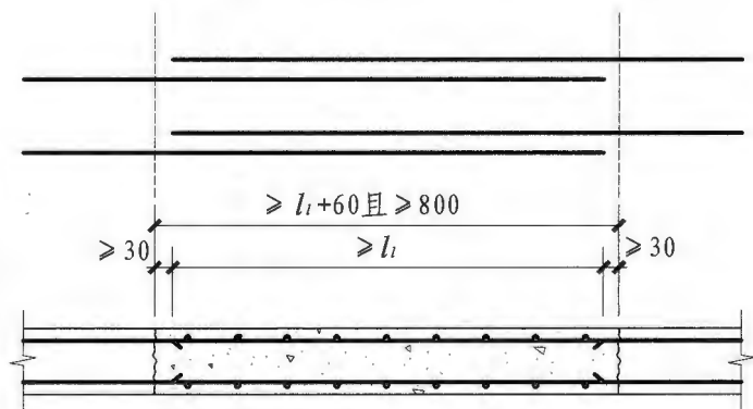
板后浇带HJD100%搭接钢筋构造
