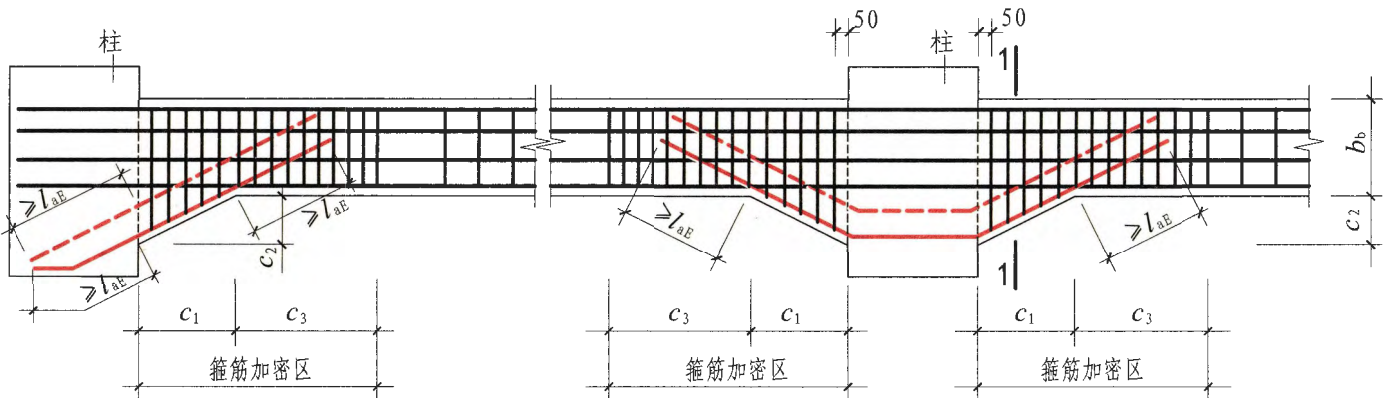
框架梁水平加腋构造
