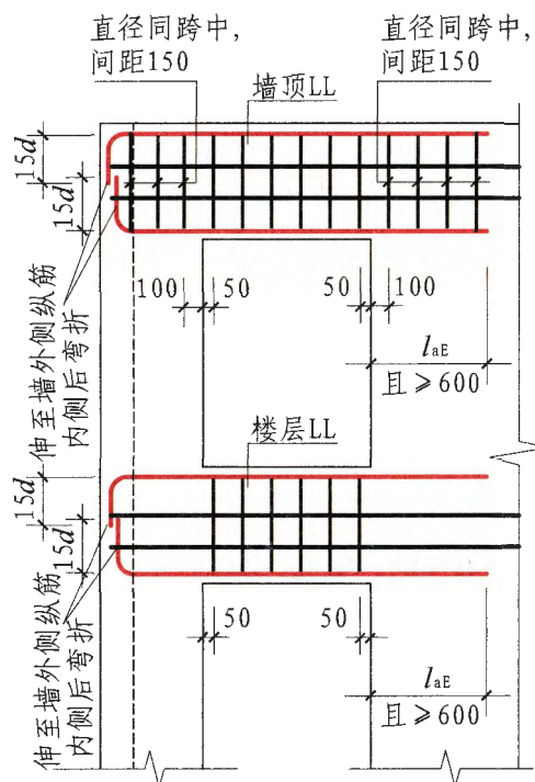
小墙垛处洞口连梁 (端部墙肢较短)
