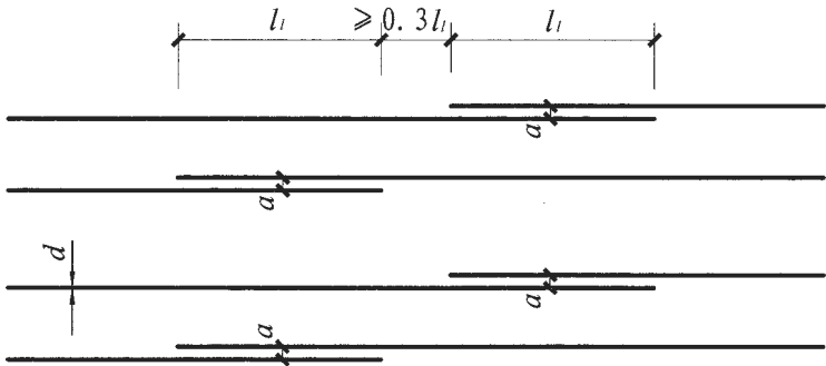
( 30+d \leq a < 0.2l_l 及150的较小值) 纵向钢筋非接触搭接构造
