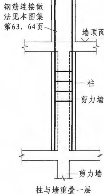
剪力墙上柱QZ纵筋构造
