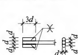
(d) 末端两侧贴焊锚筋
