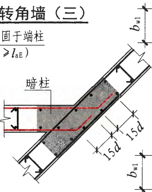
斜交翼墙
