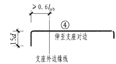
悬挑板阳角放射筋Ces构造 (本图未表示构造筋或分布筋)
