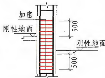
底层刚性地面前后上下各加密500
