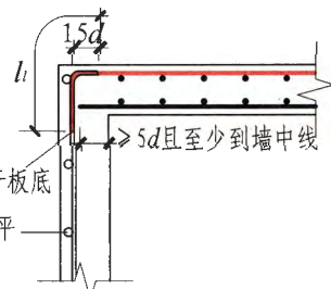
(c) 搭接连接
