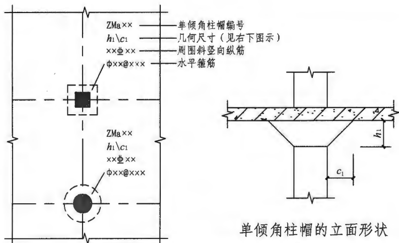
图 7.2.3-1 单倾角柱帽 ZMa 引注图示
