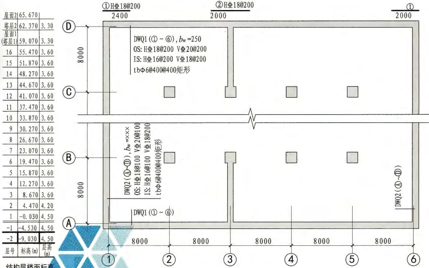
-9.030~-4.530地下室外墙平法施工图
